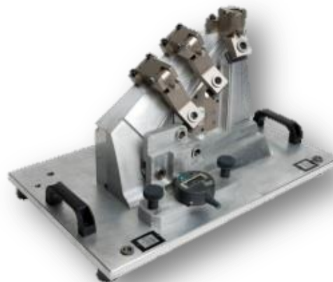
Đồ gá gia công
